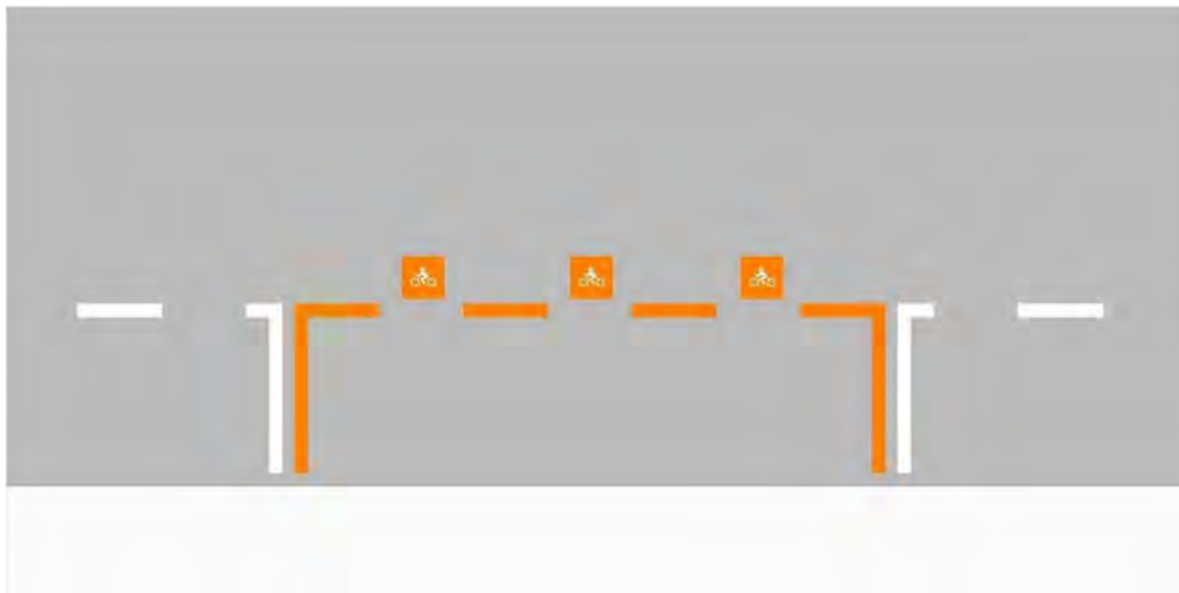
RESERVA DE MOTOS SIN HORQUILLA INTERMEDIA
