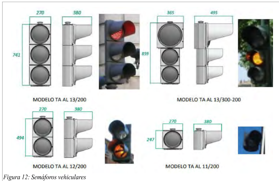
Figura 12: Semáforos vehiculares
