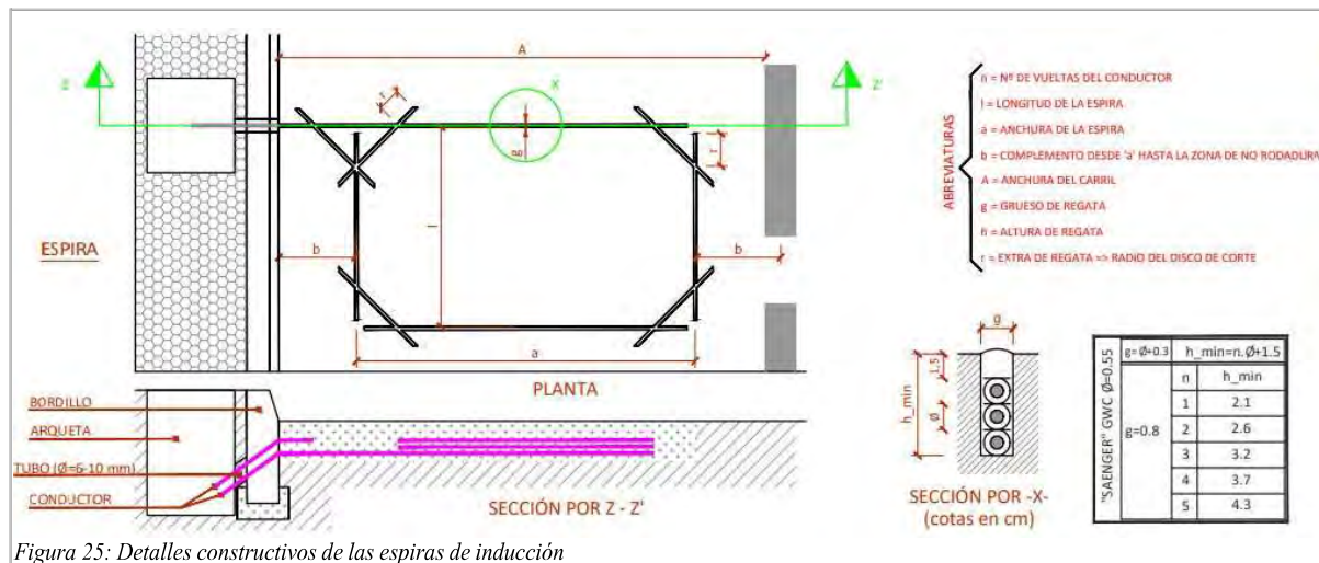
Figura 25: Detalles constructivos de las espiras de inducción
