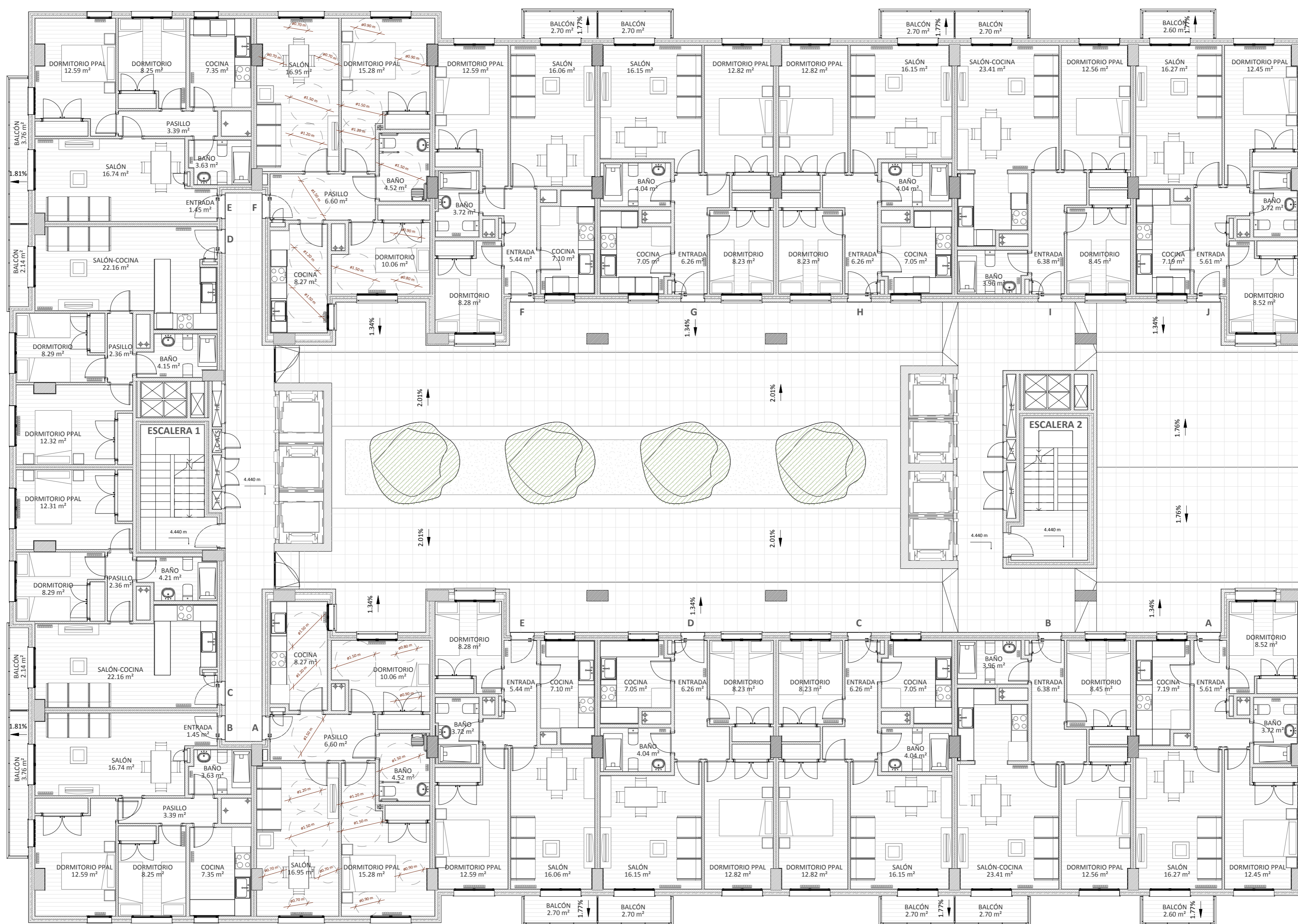
PLANTA PRIMERA
