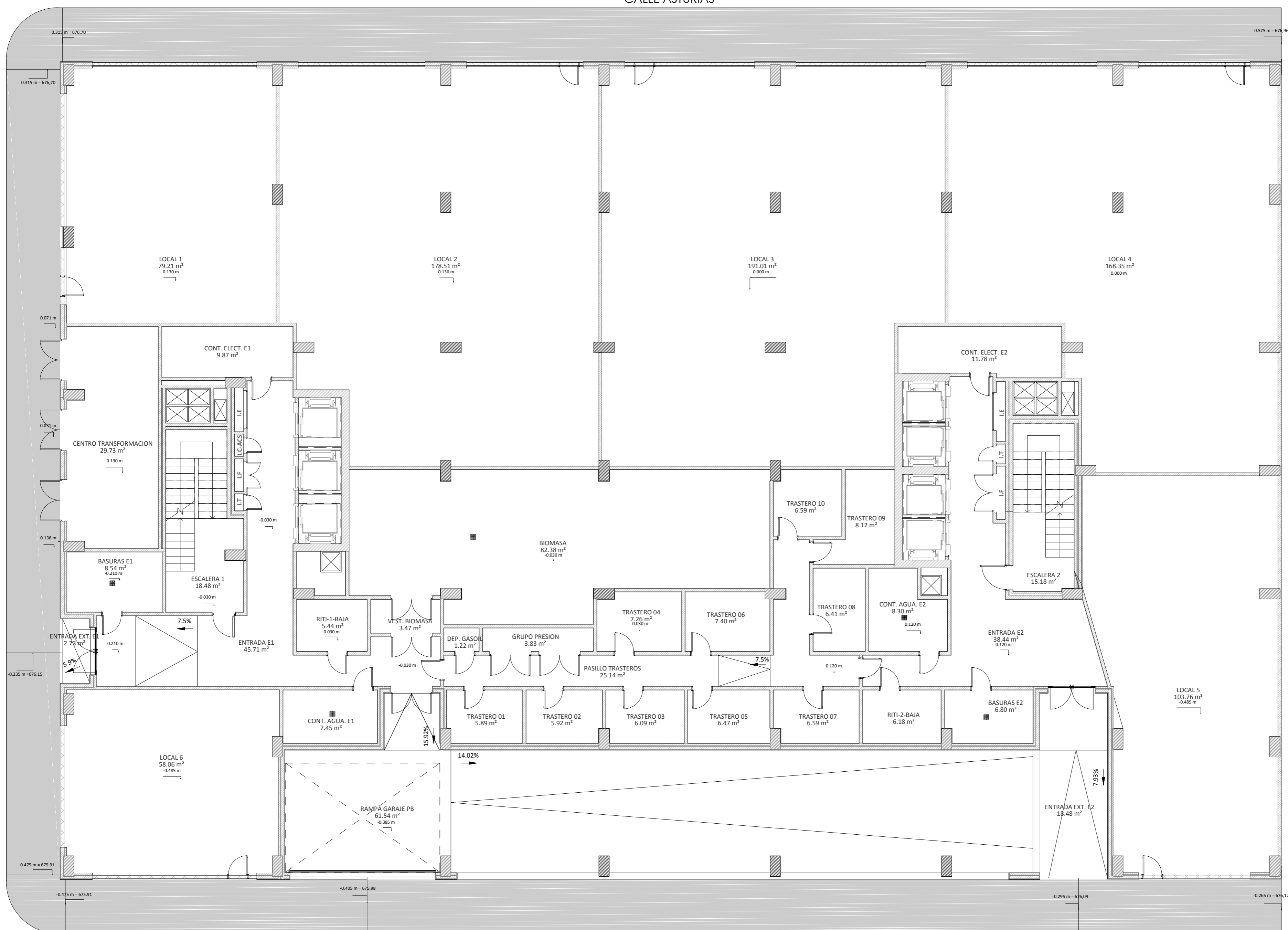
PLANTA BAJA
