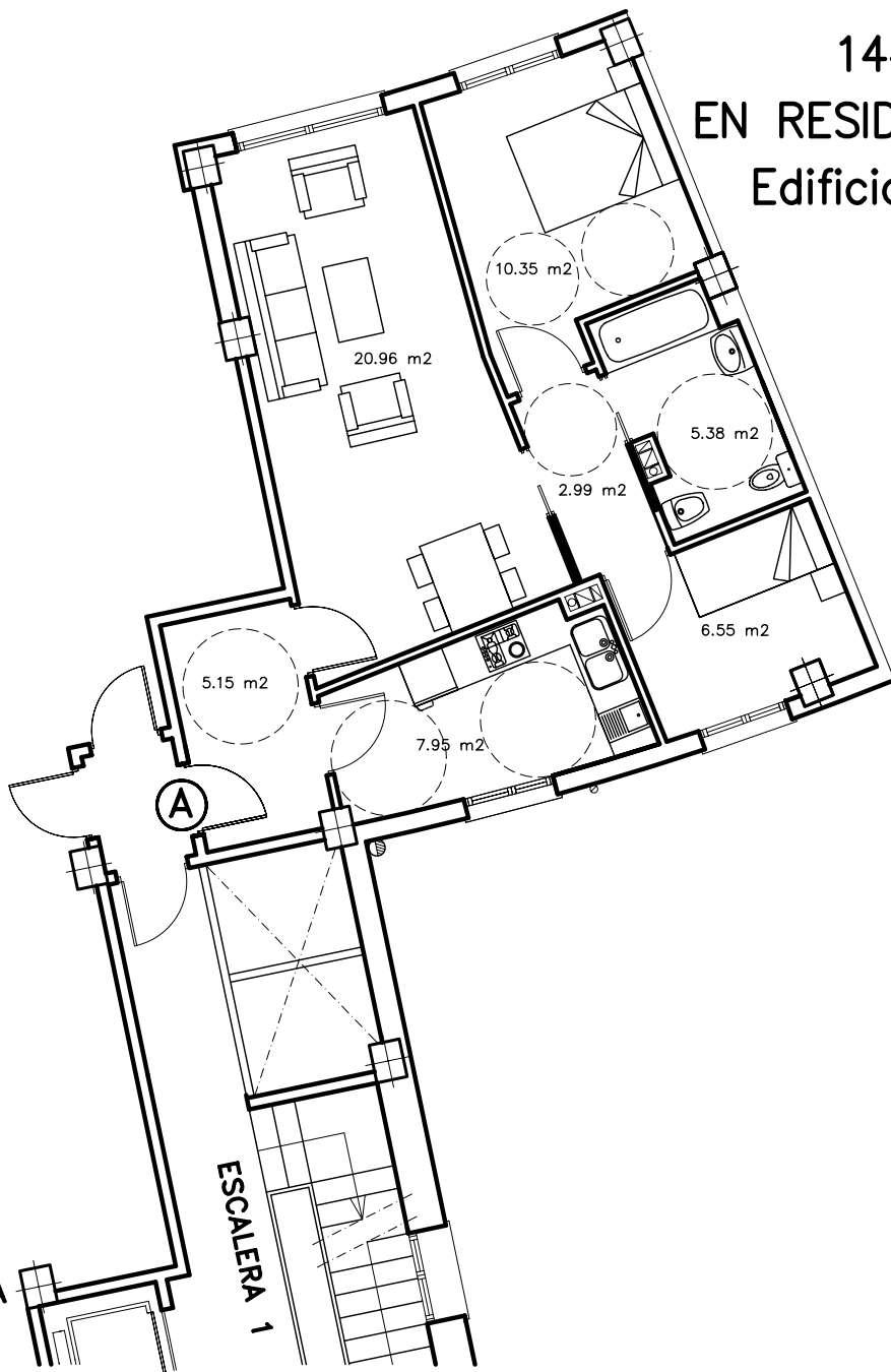
PLANTA VIVIENDA
